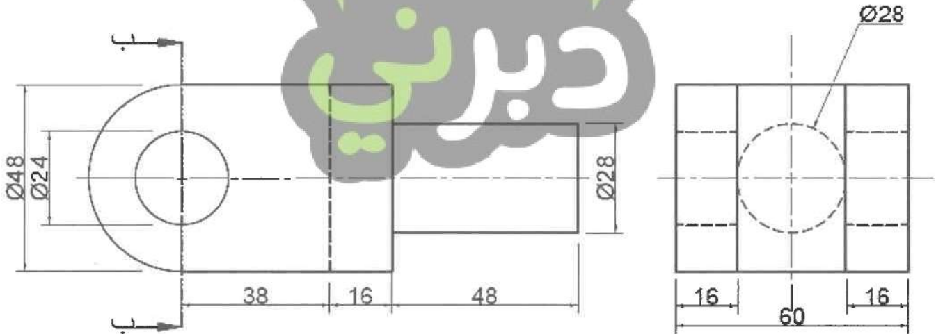
المسقط الجانبي
